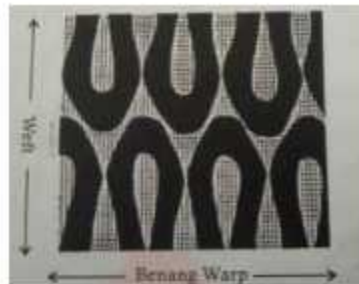
Gambar 8. Sistem Pemotongan weft system Sumber: Basuki 2014
